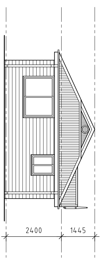
E SIDE ELEVATION 1:50
