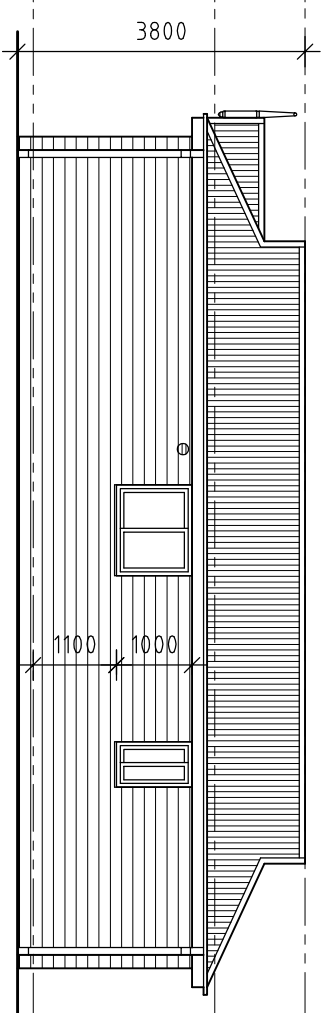
D SIDE ELEVATION 1:50
